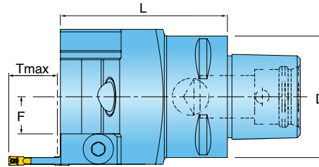
Face Groove Turn
