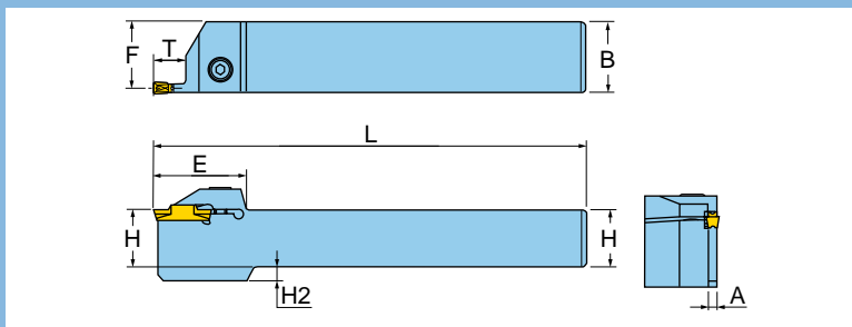
OD Profiling
