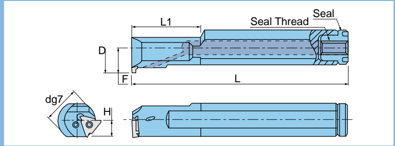
ID Grooving
