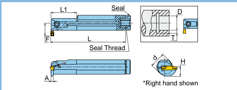
ID Profiling
