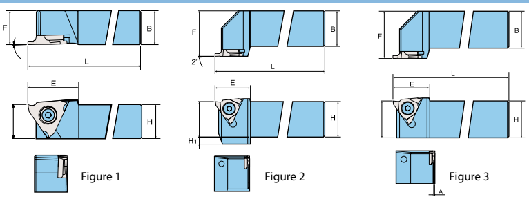
OD Grooving
