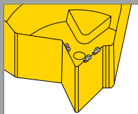
Built-up edge
