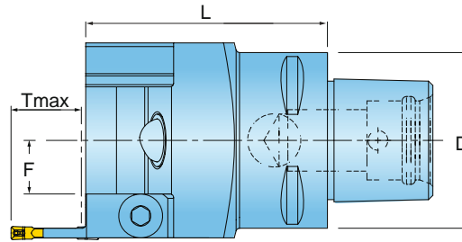
Face Groove Turn
