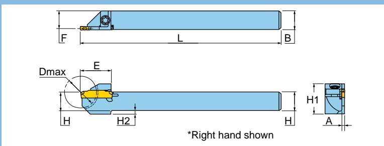
OD Profiling
